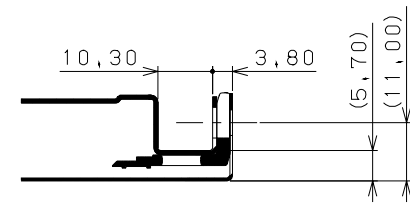
Detail J' -J'
